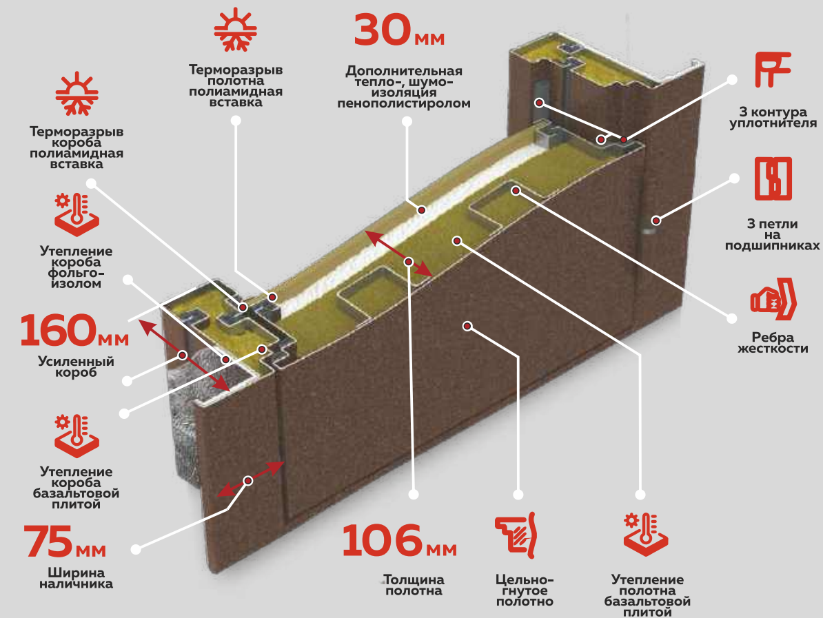
Схема дверного блока
