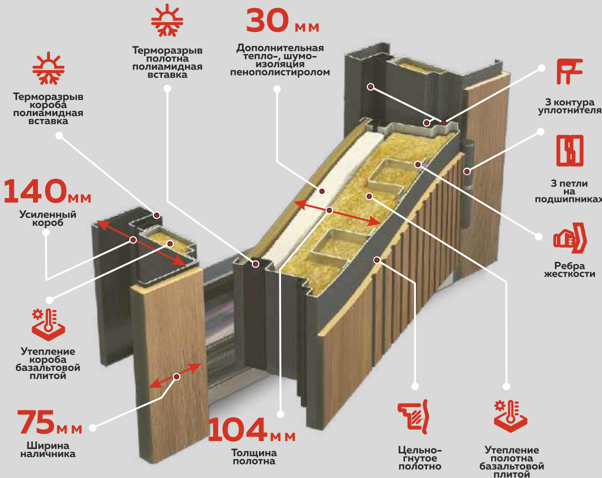
Схема дверного блока
